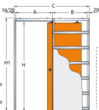
SCHEMA DE PLACEMENT DES ÉLÉMENTS EXTENSIBLES DU DORMANT POUR SYSTÈME COULISSANT DISSIMULÉ DANS LE MUR
