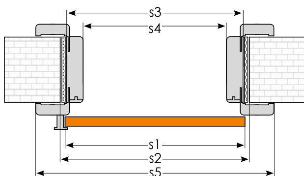
DIMENSIONS DU VANTAIL ET DU CADRE DE MUR POUR SYSTÈME POSE MURALE (mm)
