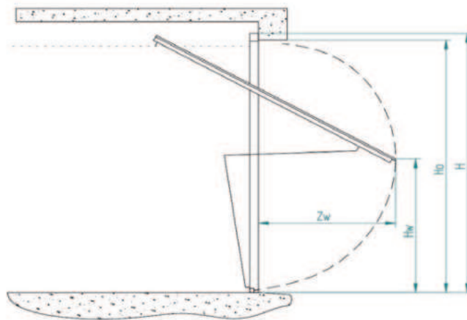
Pose derrière la baie (en applique)
